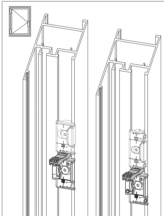
режим микровентиляция
