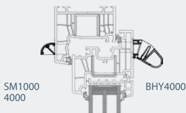
Окно ПВХ
